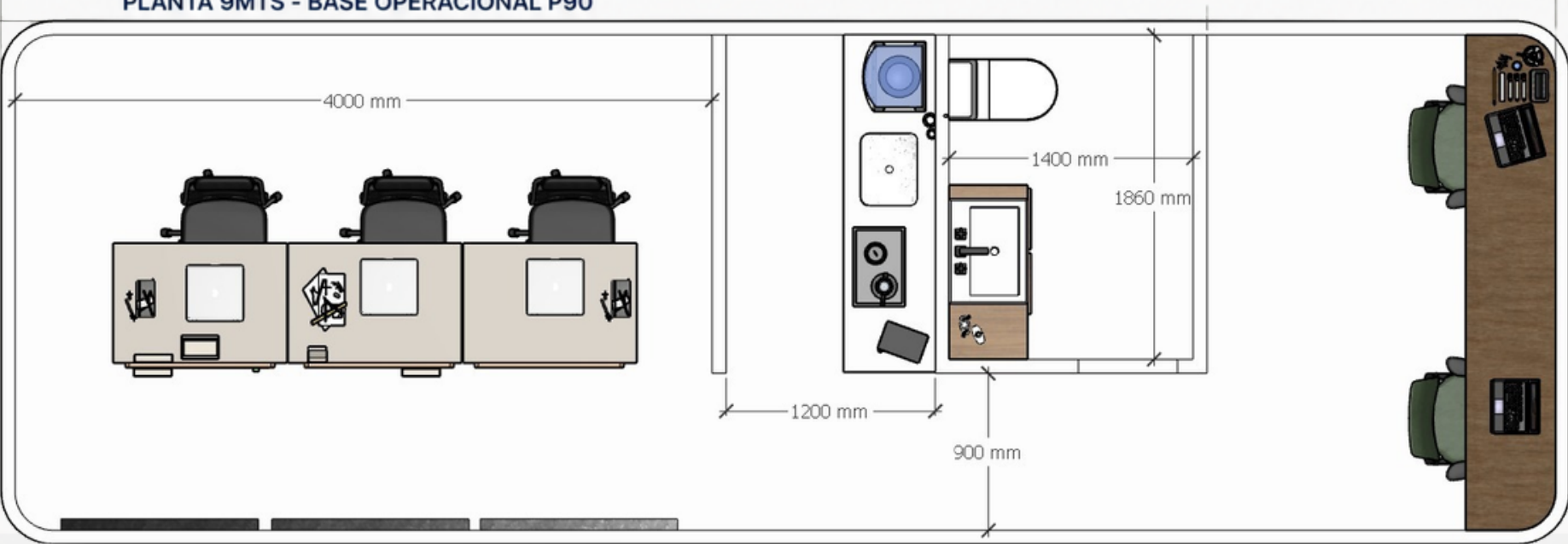
PLANTA 9MTS - BASE OPERACIONAL P90
